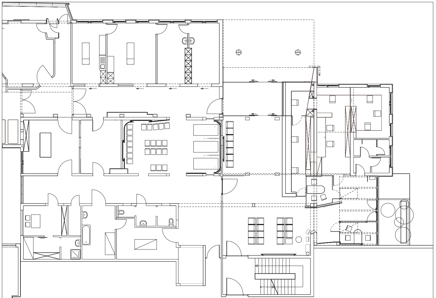
Grundriss
